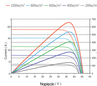
Charakterystyka prądowo – napięciowa (665W)
